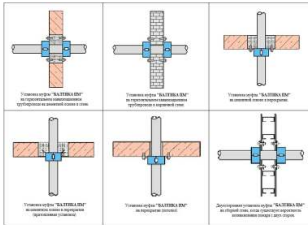
Схема установки 1
